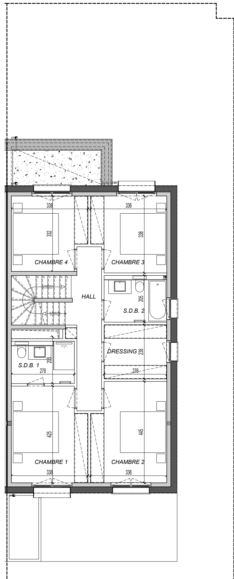
ETAGE 1/100
