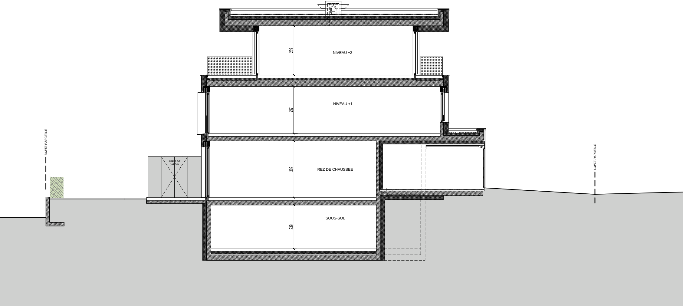
COUPE 1/100
