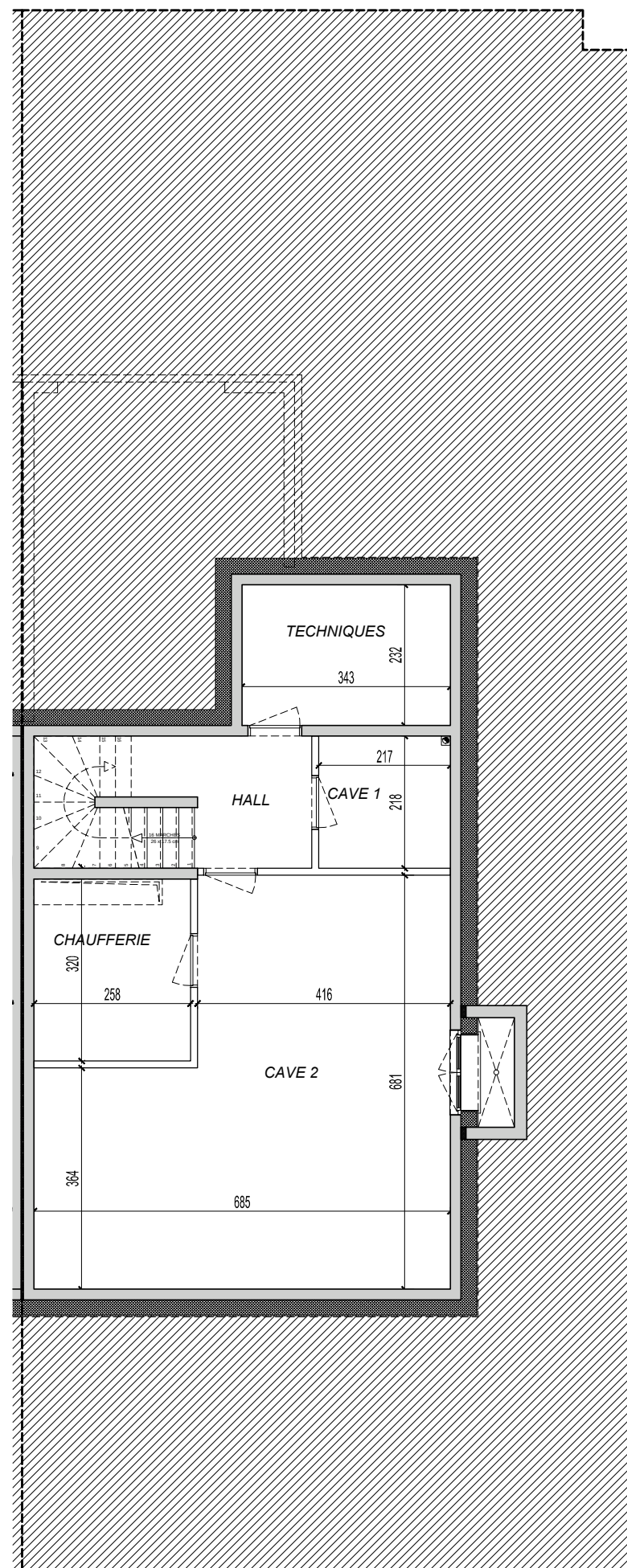
SOUS-SOL 1/100
