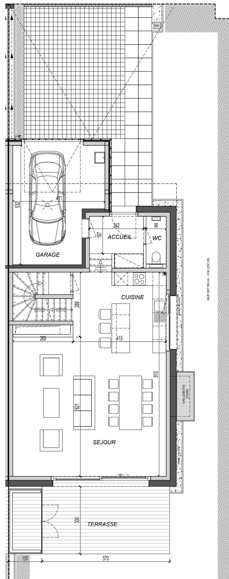
REZ-DE-CHAUSSEE 1/100
